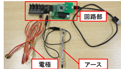
図2 筋電位計測デバイス
