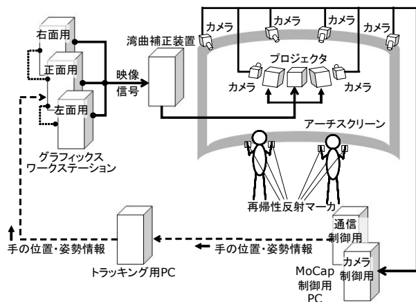
図2 システム構成 Fig. 2 Hardware system configurations
